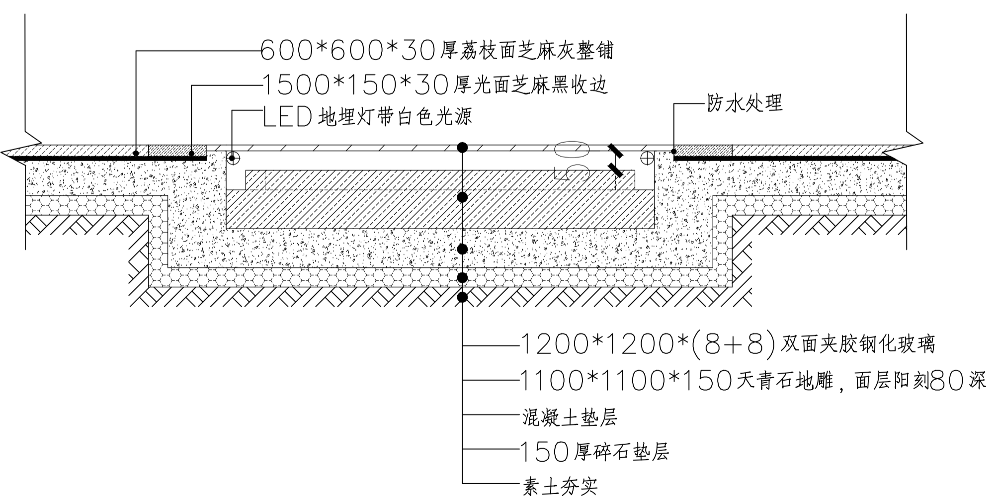
1-1 剖
